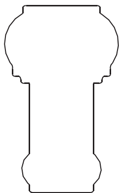
Överliggare Nr.H1 120x73mm Herrgård
